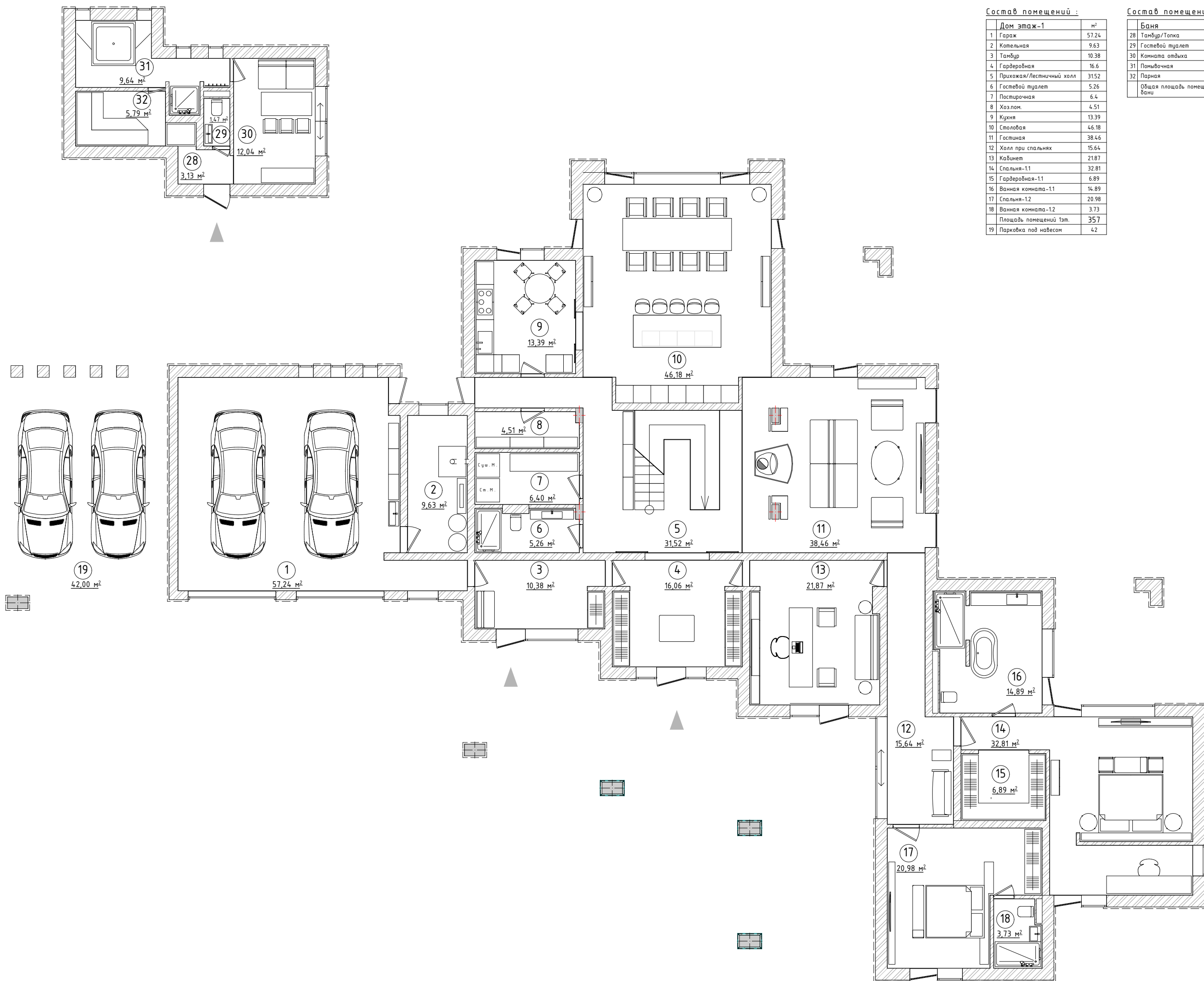
Состав помещений :
