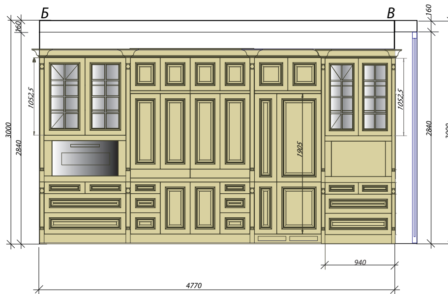
Схема №2.8.7. Схема развертки стен в помещении кухни с примеркой материалов
