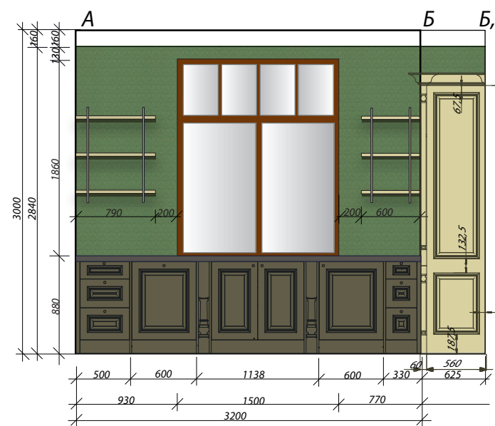
Схема №2.8.7. Схема развертки стен в помещении кухни с примеркой материалов
