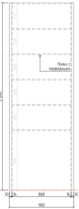
ВНУТРЕННЕЕ НАПОЛНЕНИЕ
