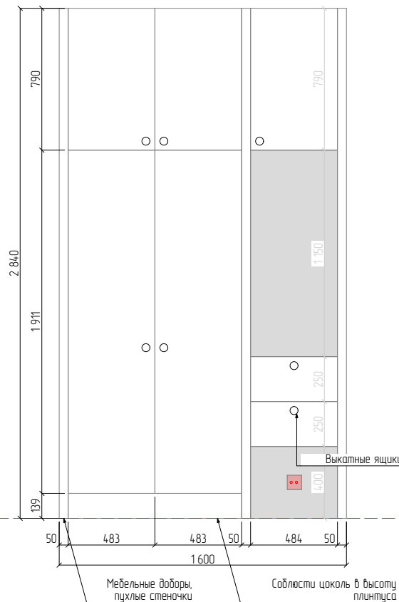
ФАСАД
