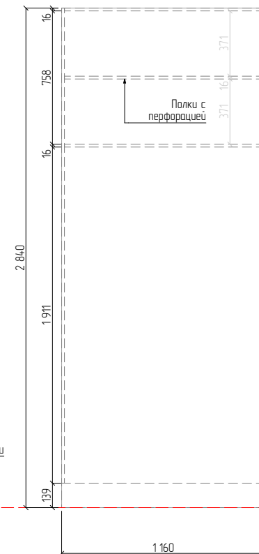
ВНУТРЕННЕЕ НАПОЛНЕНИЕ
