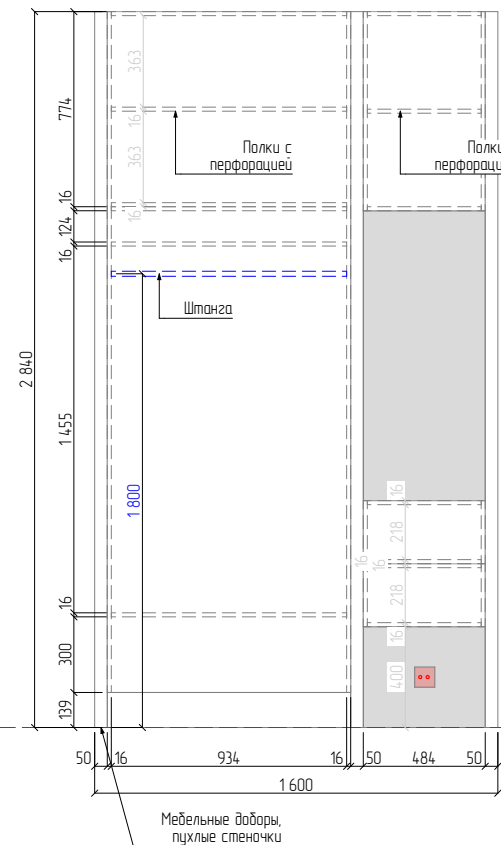
ВНУТРЕННЕЕ НАПОЛНЕНИЕ
