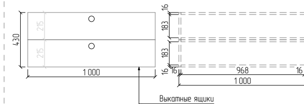
ФАСАД
