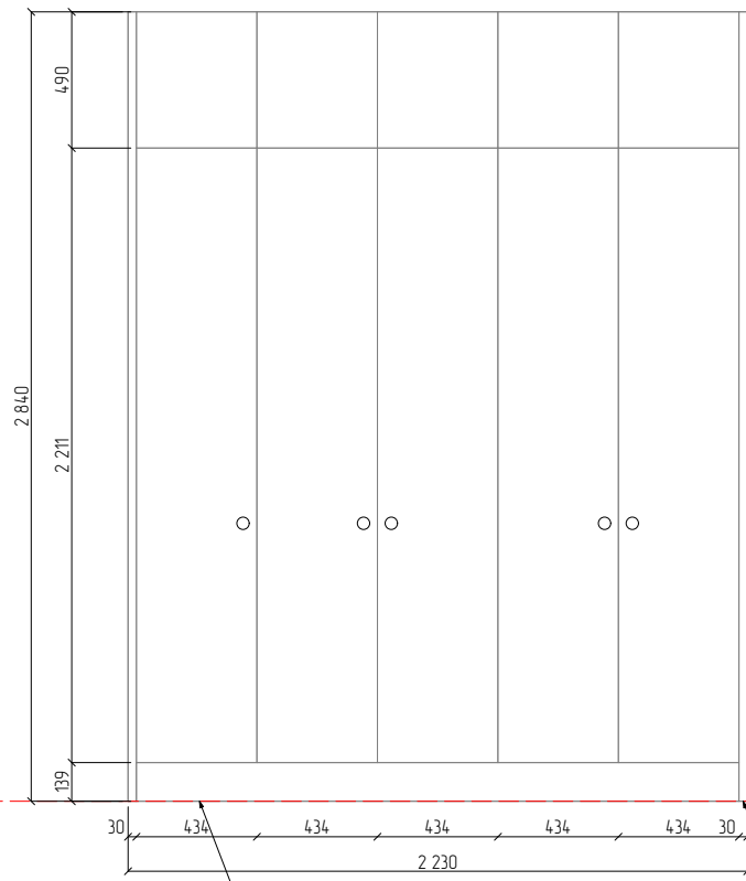
ФАСАД
