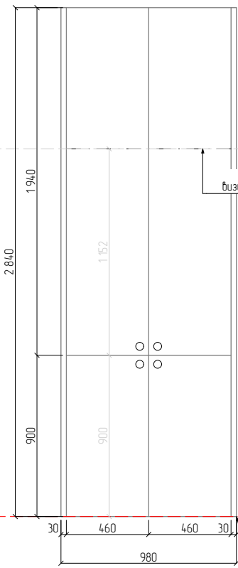
ФАСАД
