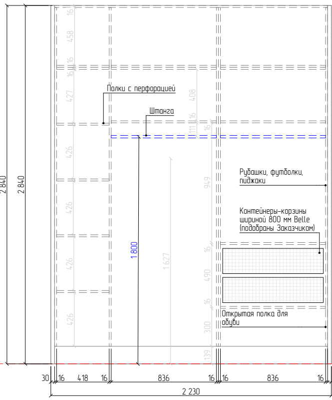
ВНУТРЕННЕЕ НАПОЛНЕНИЕ
