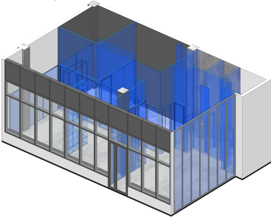
Общая аксонометрия
