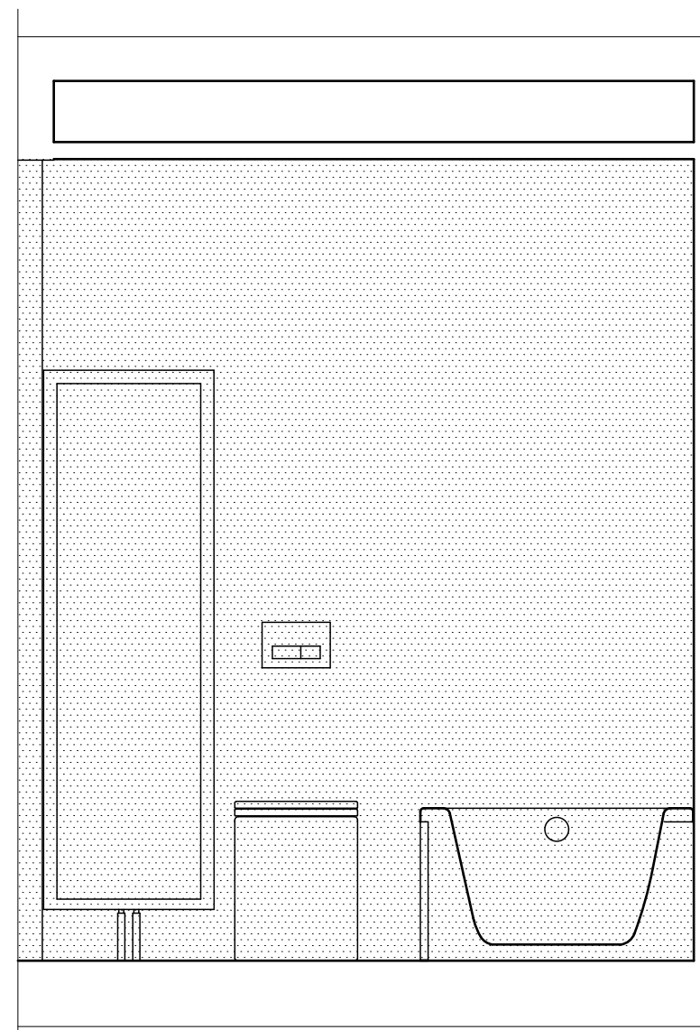
Разрез 2-2
