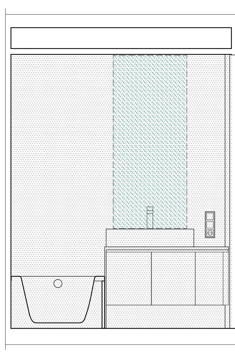
Разрез 10-10
