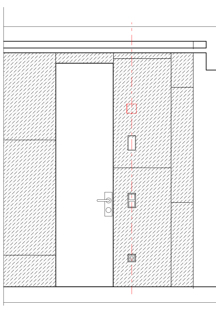
Разрез 11-11
