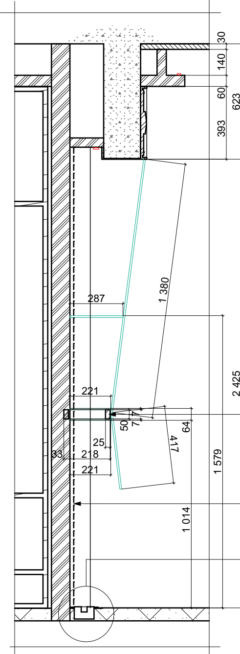
Разрез 24-24
