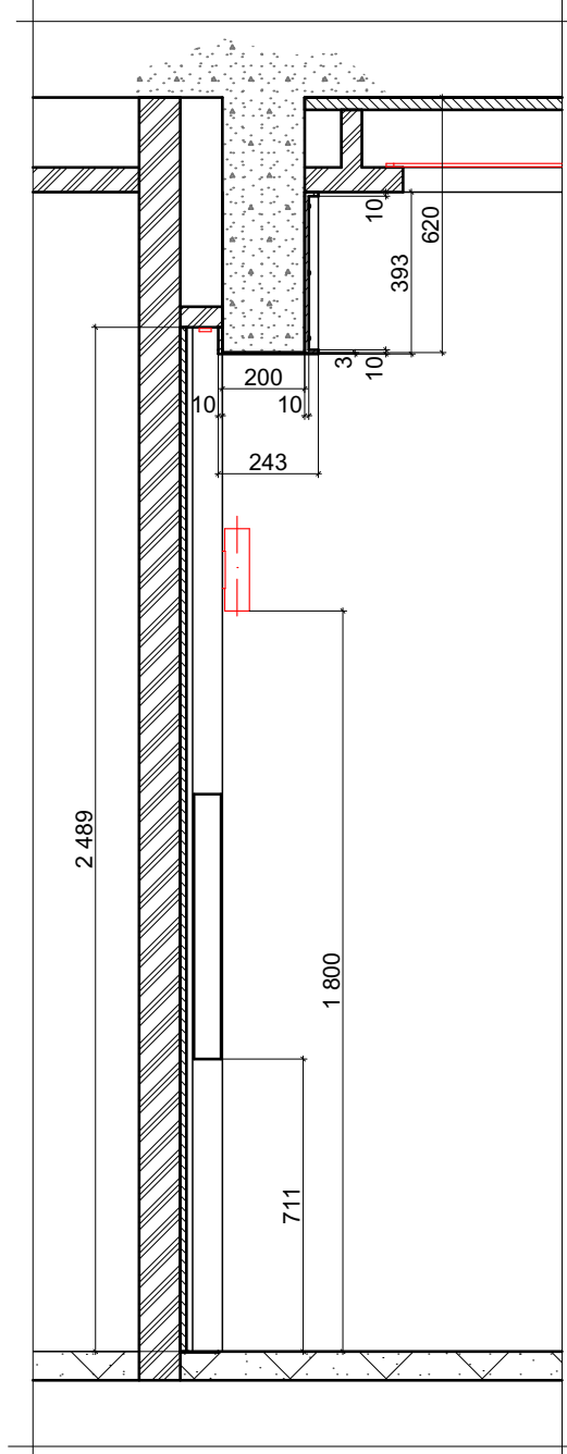
Разрез 23-23
