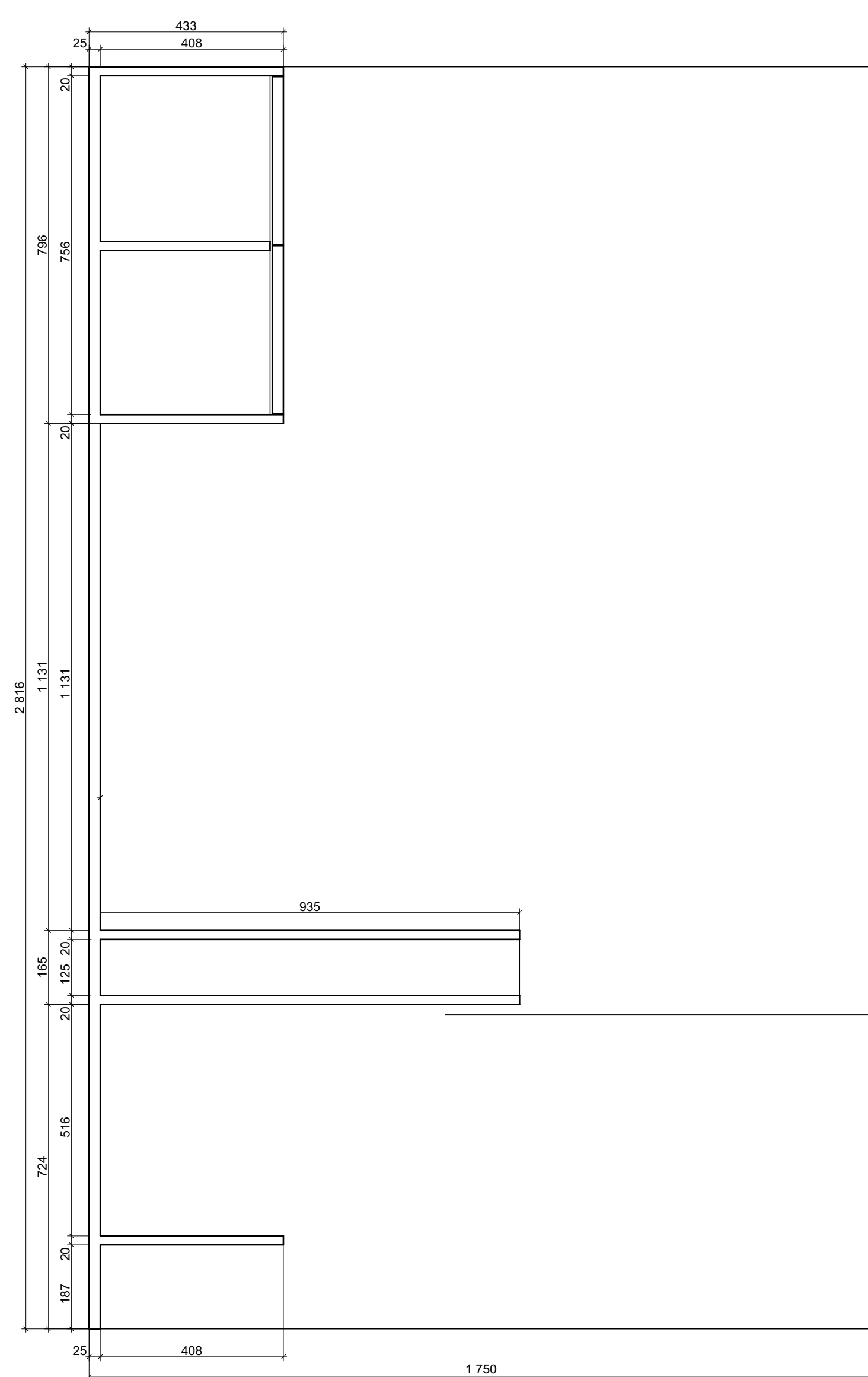
Детализация выдвижного ящика
