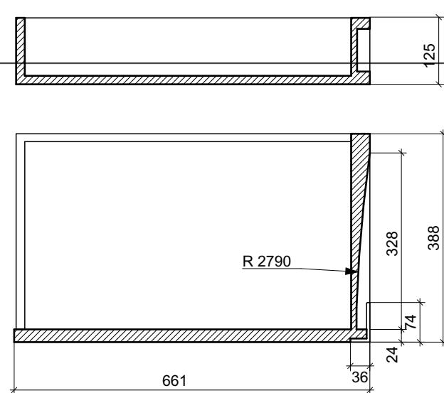
Детализация выдвижного ящика
