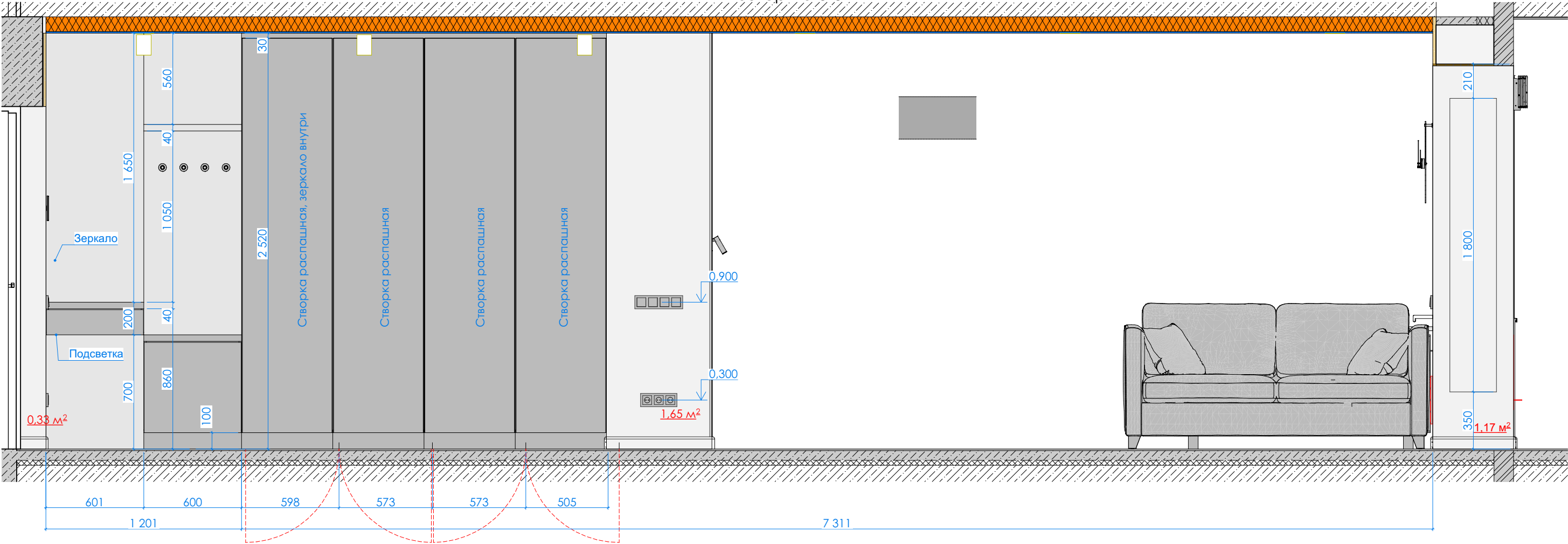
Развёртка 3-3
