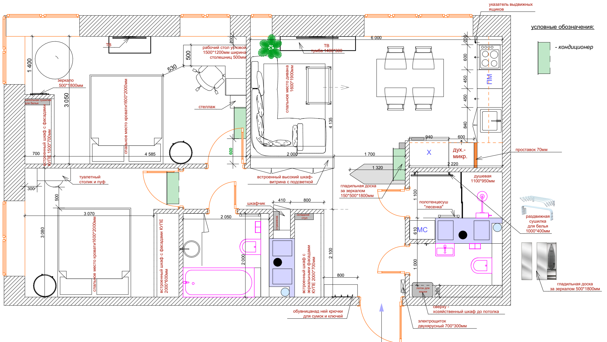
План с размещением мебели, сантехники и кондиционеров
