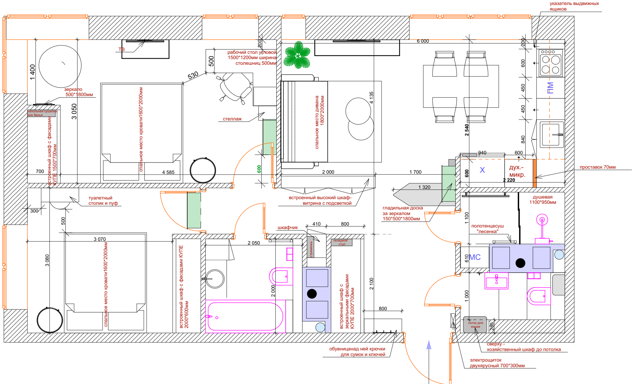
План с размещением мебели, сантехники и кондиционеров
